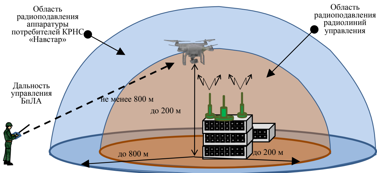
Рис. 13. Вариант применения станции помех РП-377УВМ1Л «Лесочек», при РЭП радиопередачи управления и аппаратуры потребителей КРНС БпЛА
