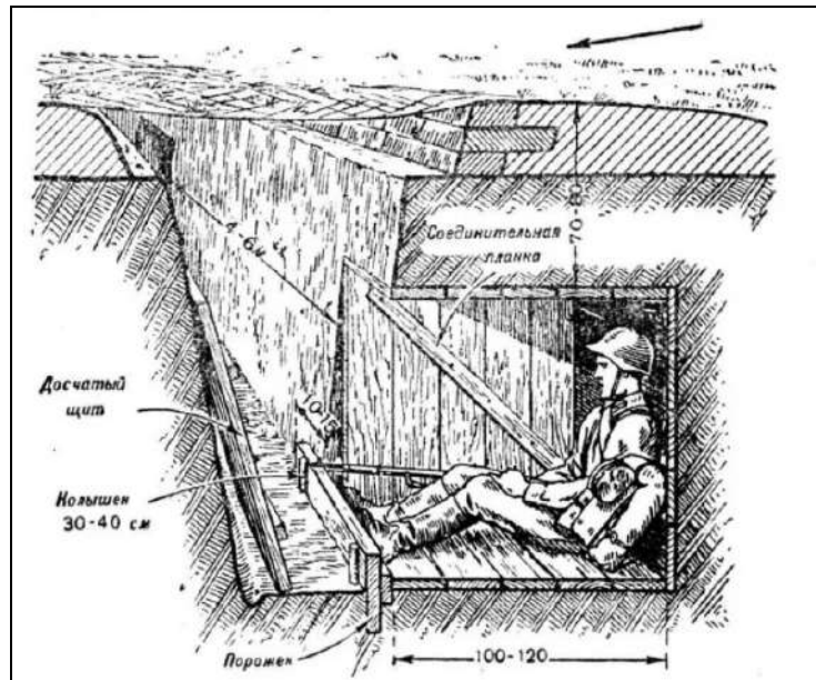
Рис. 3. Оборудование укрытия типа «Лисья нора»
